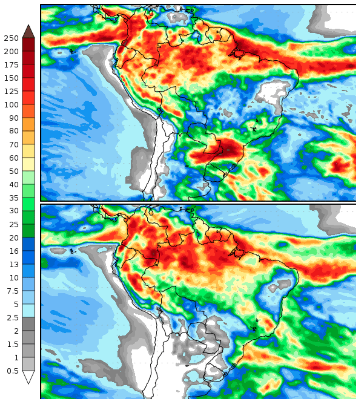
Figura 1. Acumulados de precipitação previstos entre os dias 07 e 15 de abril (imagem superior) e 15 e 23 de abril de 2022 (imagem inferior). Fonte: COLA (Center for Ocean-Land-Atmosphere-Studies).
