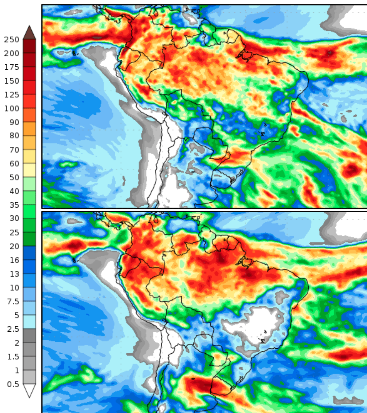
Figura 1. Acumulados de precipitação previstos entre os dias 11 e 19 de abril (imagem superior) e 19 e 27 de abril de 2022 (imagem inferior). Fonte: COLA (Center for Ocean-Land-Atmosphere-Studies).
