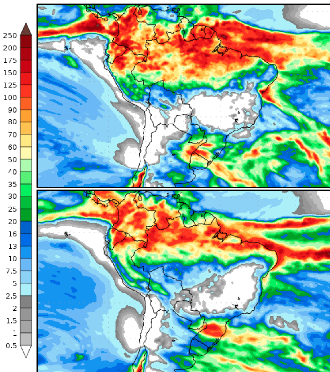
Figura 1. Acumulados de precipitação previstos entre os dias 18 e 26 de abril (imagem superior) e 26 de abril a 04 de maio de 2022 (imagem inferior). Fonte: COLA (Center for Ocean-Land-Atmosphere-Studies).
