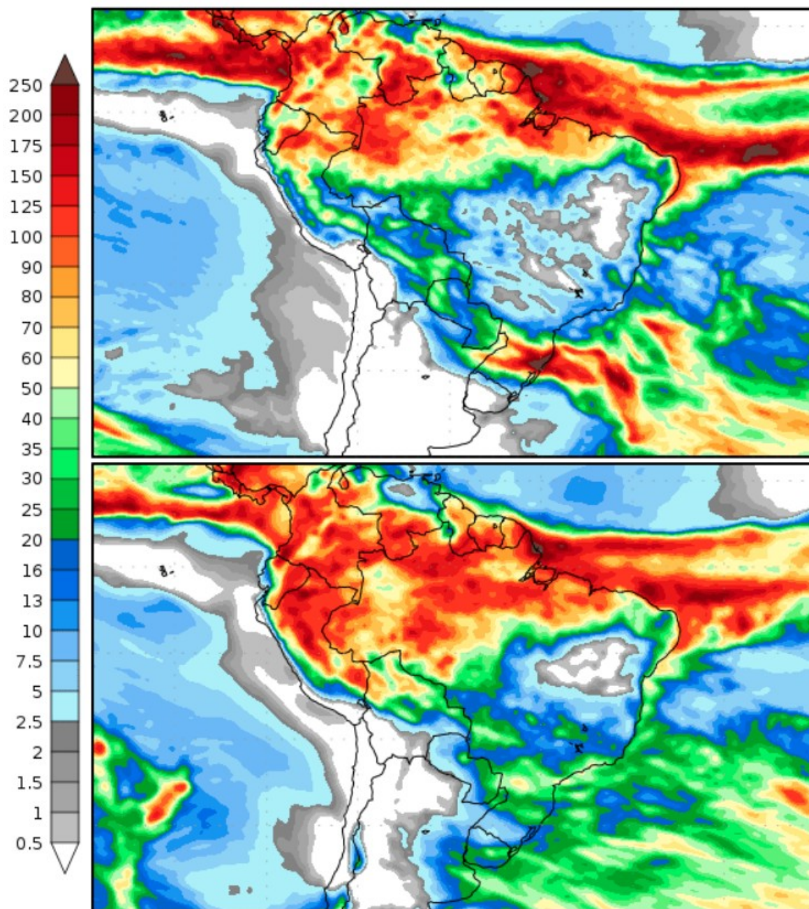
Figura 1. Acumulados de precipitação previstos entre os dias 02 a 10 de maio (imagem superior) e 10 a 18 de maio de 2022 (imagem inferior). Fonte: COLA (Center for Ocean-Land-Atmosphere-Studies).
