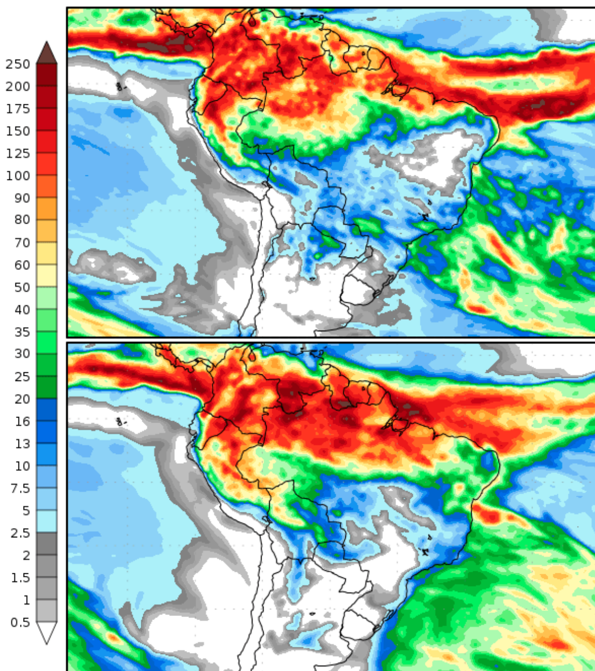
Figura 1. Acumulados de precipitação previstos entre os dias 05 a 13 de maio (imagem superior) e 13 a 21 de maio de 2022 (imagem inferior). Fonte: COLA (Center for Ocean-Land-Atmosphere-Studies).
