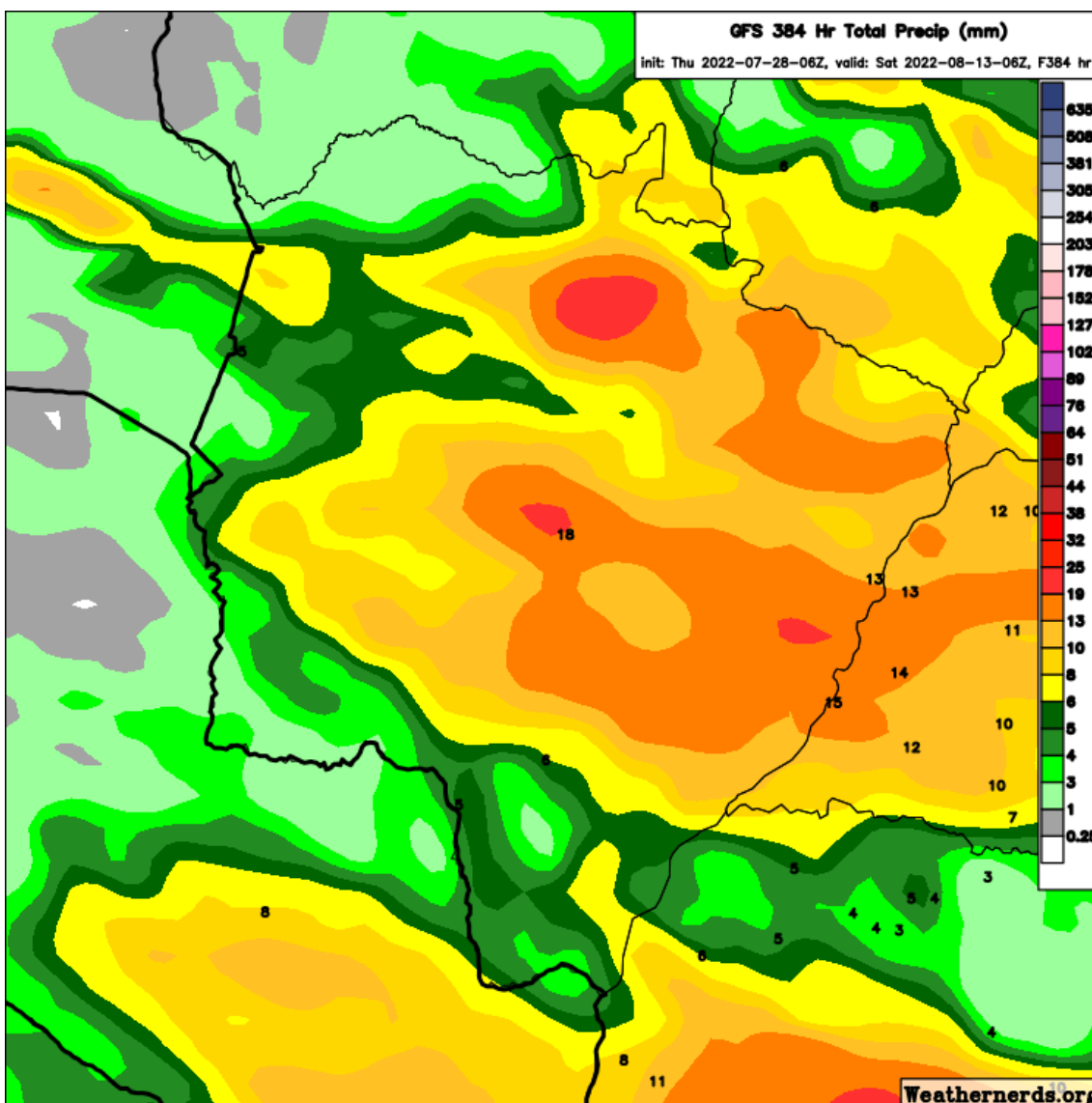
Figura 1. Precipitação acumulada prevista entre os dias 28 de julho a 13 de agosto de 2022. Fonte: Modelo GFS/tropicaltidbits.com.
