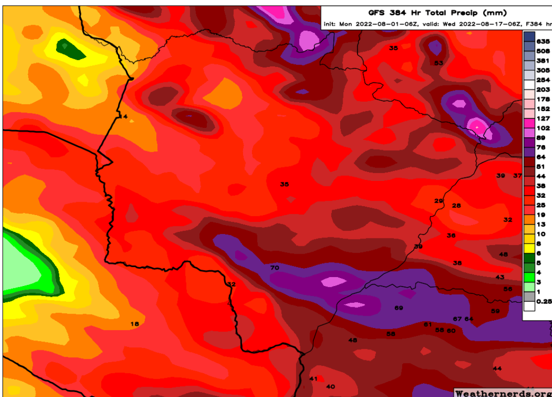
Figura 1. Precipitação acumulada prevista entre os dias 01 a 17 de agosto de 2022. Fonte: Modelo GFS/Weathernerds.
