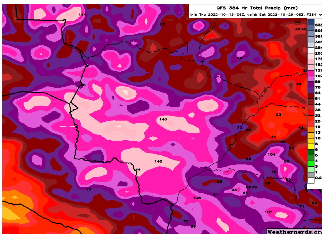
Figura 1. Precipitação acumulada prevista entre os dias 13 a 29 de outubro de 2022. Fonte: Modelo GFS/Weathernerds.
