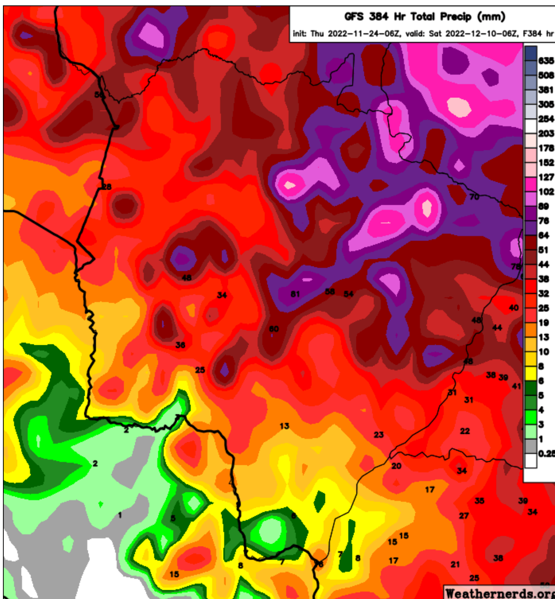
Figura 1. Precipitação acumulada prevista entre os dias 24 de novembro a 10 de dezembro de 2022. Fonte: Modelo GFS/Weathernerds.
