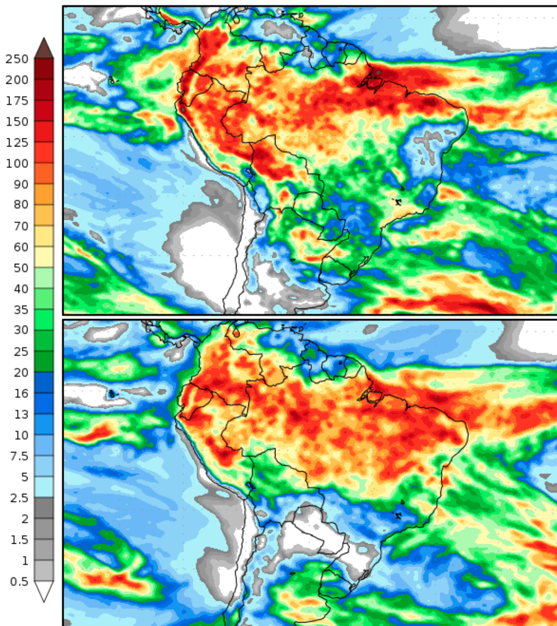
Figura 1. Precipitação acumulada prevista entre os dias 30 de março a 07 de abril de 2023 (a) e 07 a 15 de abril de 2023 (b). Fonte: Modelo GFS.
