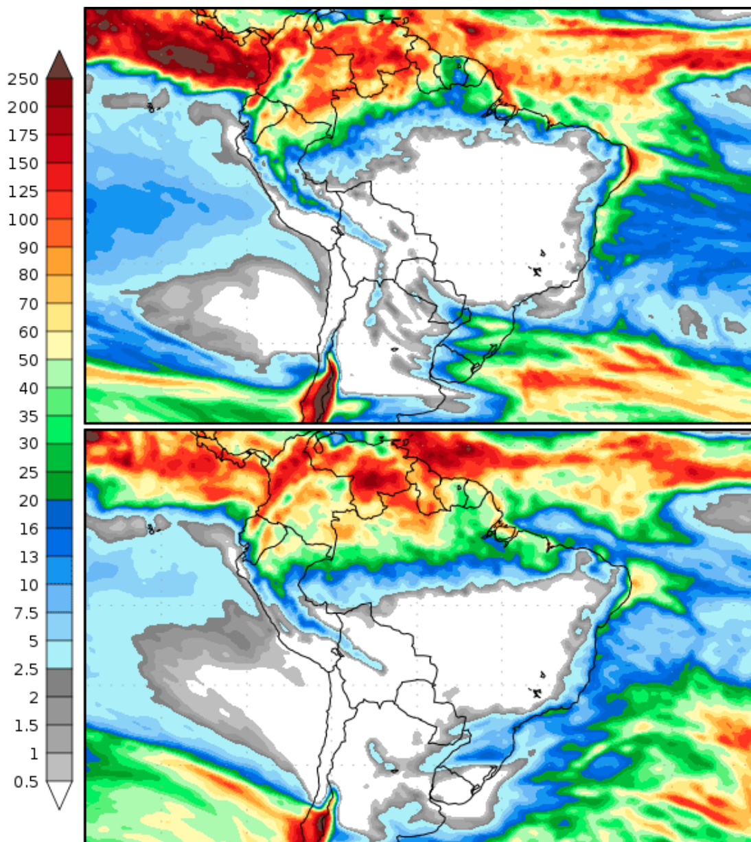
Figura 1. Precipitação acumulada prevista entre os dias 22 a 30 de junho (imagem superior) e 30 de junho a 08 de julho de 2023 (imagem inferior). Fonte: COLA (Center for Ocean-Land-Atmosphere-Studies).
