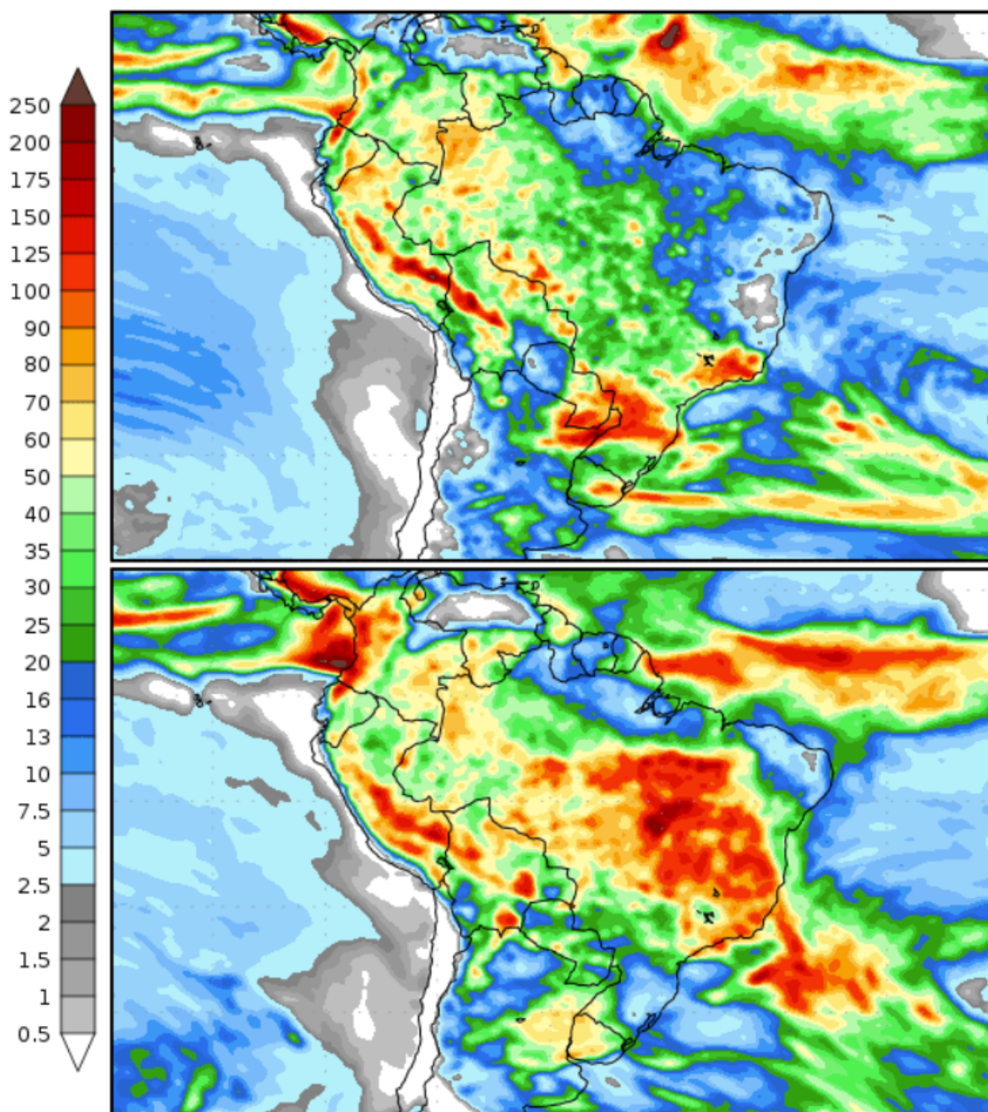
Figura 1. Precipitação acumulada prevista entre os dias 04 a 12 de dezembro (imagem superior) e 12 a 20 de dezembro de 2023 (imagem inferior). Fonte: COLA (Center for Ocean-Land-Atmosphere-Studies).
