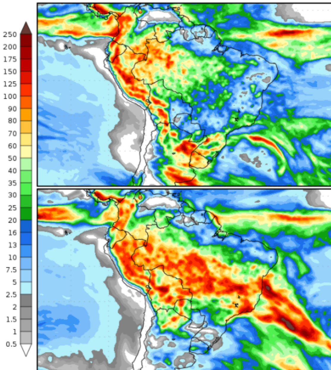
Figura 1. Precipitação acumulada prevista entre os dias 11 a 19 de dezembro (imagem superior) e 19 a 27 de dezembro de 2023 (imagem inferior). Fonte: COLA (Center for Ocean-Land-Atmosphere-Studies).
