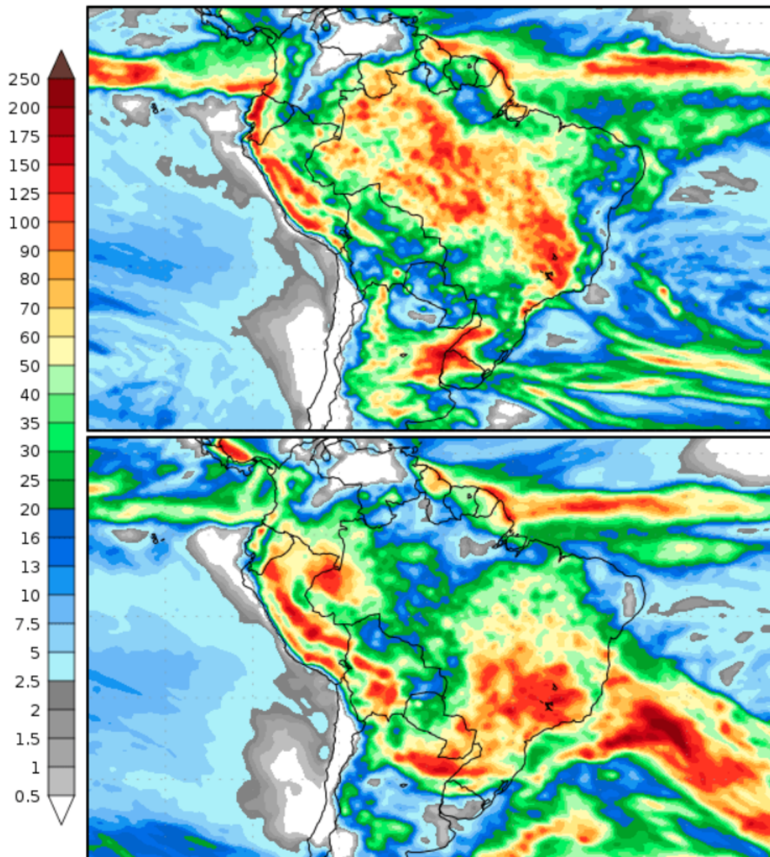
Figura 1. Precipitação acumulada prevista entre os dias 08 a 16 de janeiro (imagem superior) e 16 a 24 de janeiro de 2024 (imagem inferior). Fonte: COLA (Center for Ocean-Land-Atmosphere-Studies).
