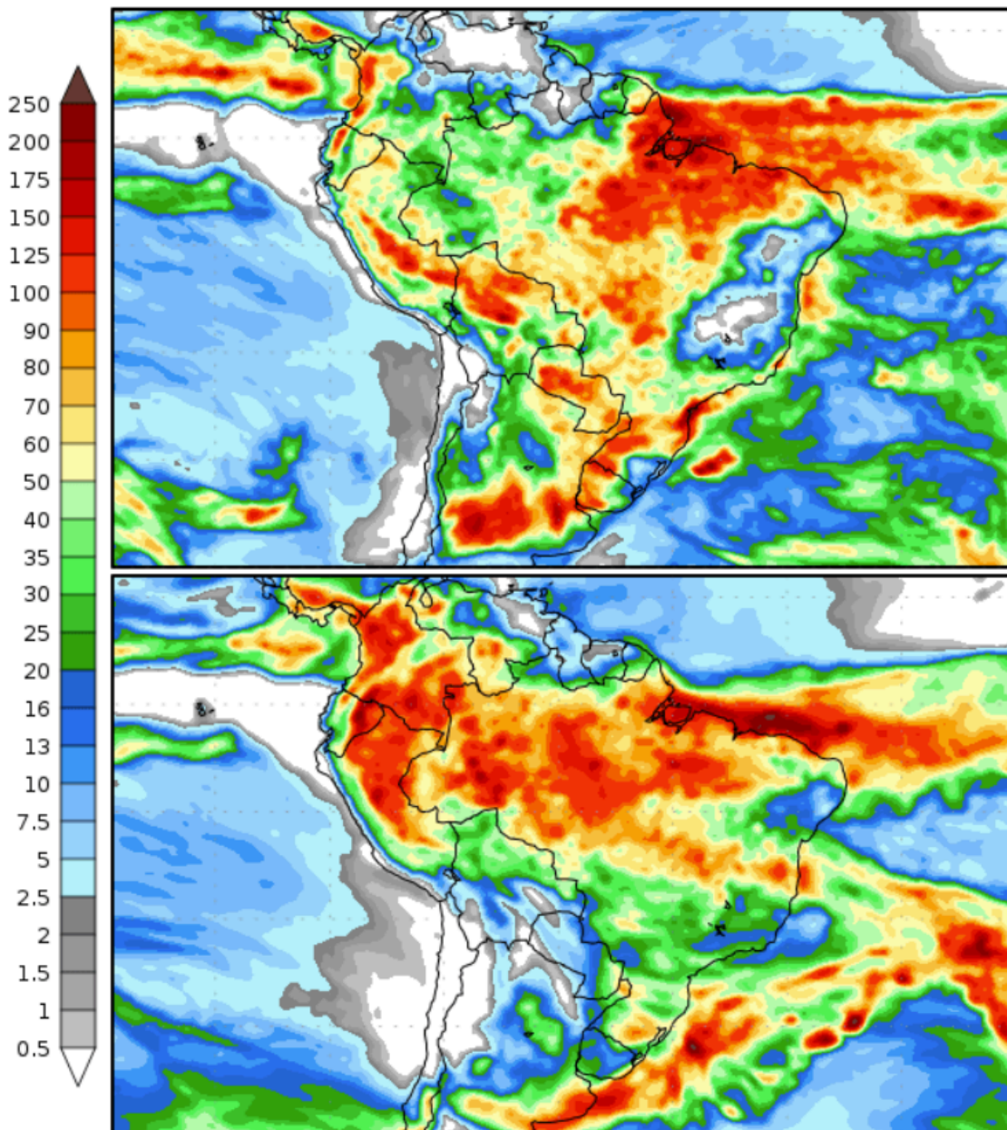
Figura 1. Precipitação acumulada prevista entre os dias 08 a 16 de abril (imagem superior) e 16 a 24 de abril de 2024 (imagem inferior). Fonte: COLA (Center for Ocean-Land-Atmosphere-Studies).
