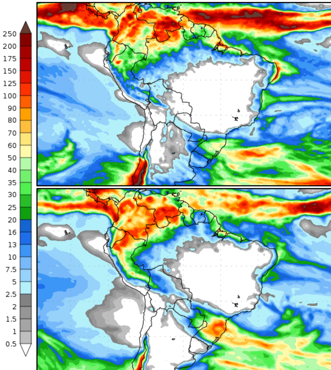
Figura 1. Precipitação acumulada prevista entre os dias 20 a 28 de junho (imagem superior) e 28 de junho a 06 de julho de 2024 (imagem inferior). Fonte: COLA (Center for Ocean-Land-Atmosphere-Studies).
