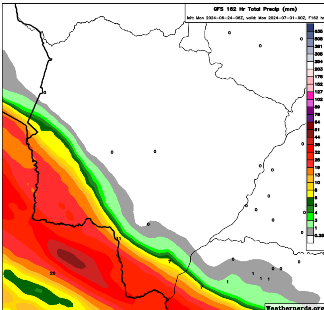
Figura 1. Precipitação acumulada prevista entre os dias 24 a 30 de junho de 2024. Fonte: Weathernerds.
