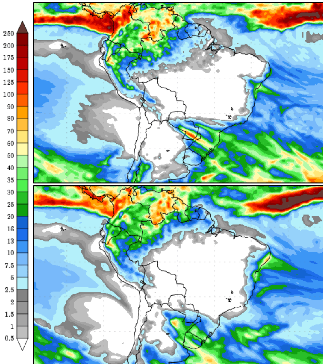
Figura 1. Precipitação acumulada prevista entre os dias 22 a 30 de agosto (imagem superior) e 30 de agosto a 07 de setembro de 2024 (imagem inferior). Fonte: COLA (Center for Ocean-Land-Atmosphere-Studies).
