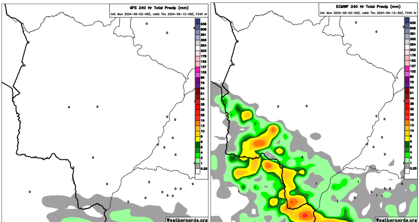
Figura 1. Precipitação acumulada prevista entre os dias 02 a 12 de setembro de 2024 a partir do modelo (a) GFS (b) ECMWF. Fonte: Weathernerds.
