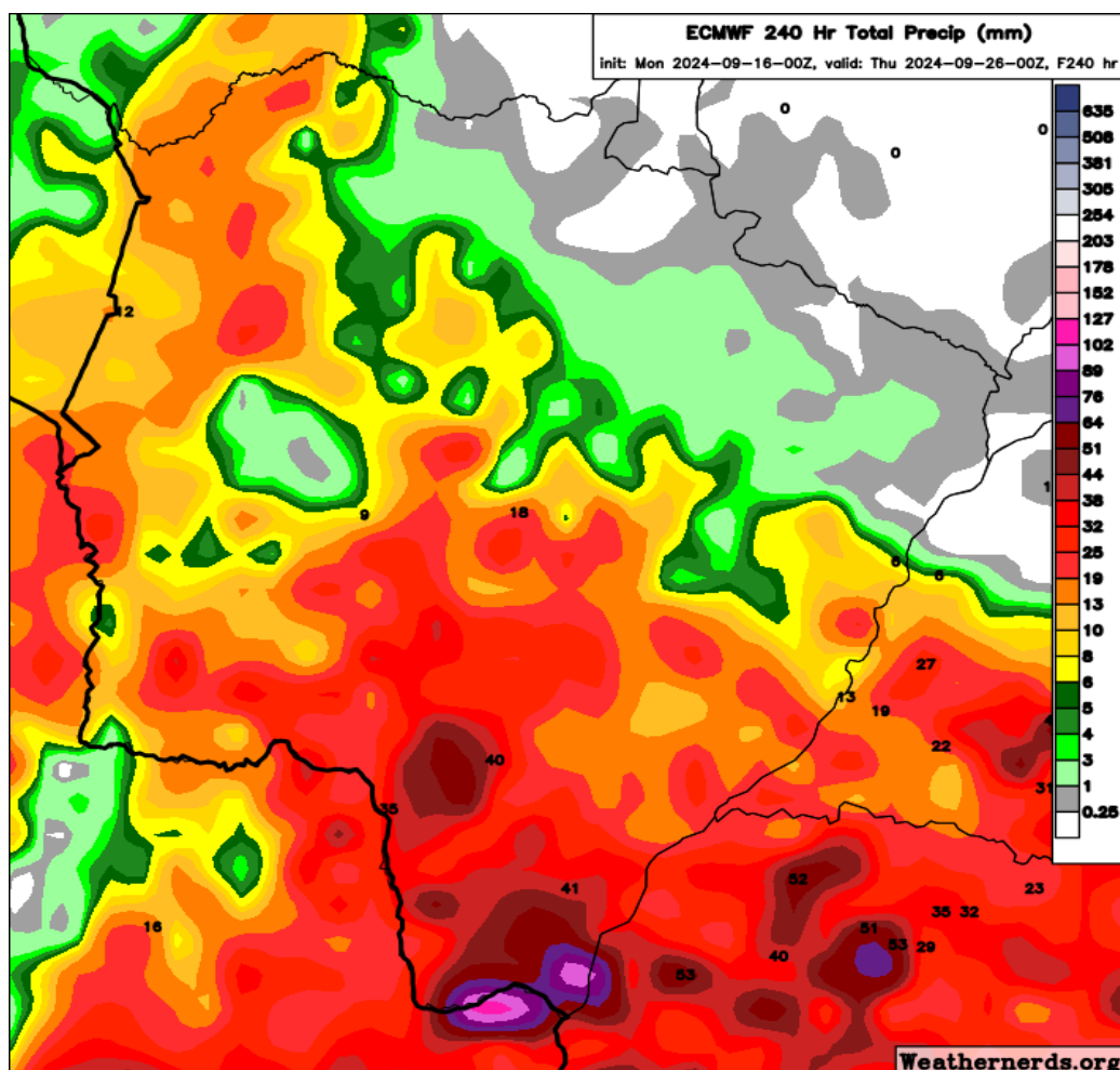
Figura 1. Precipitação acumulada prevista entre os dias 16 a 26 de setembro. Fonte: Weathernerds.
