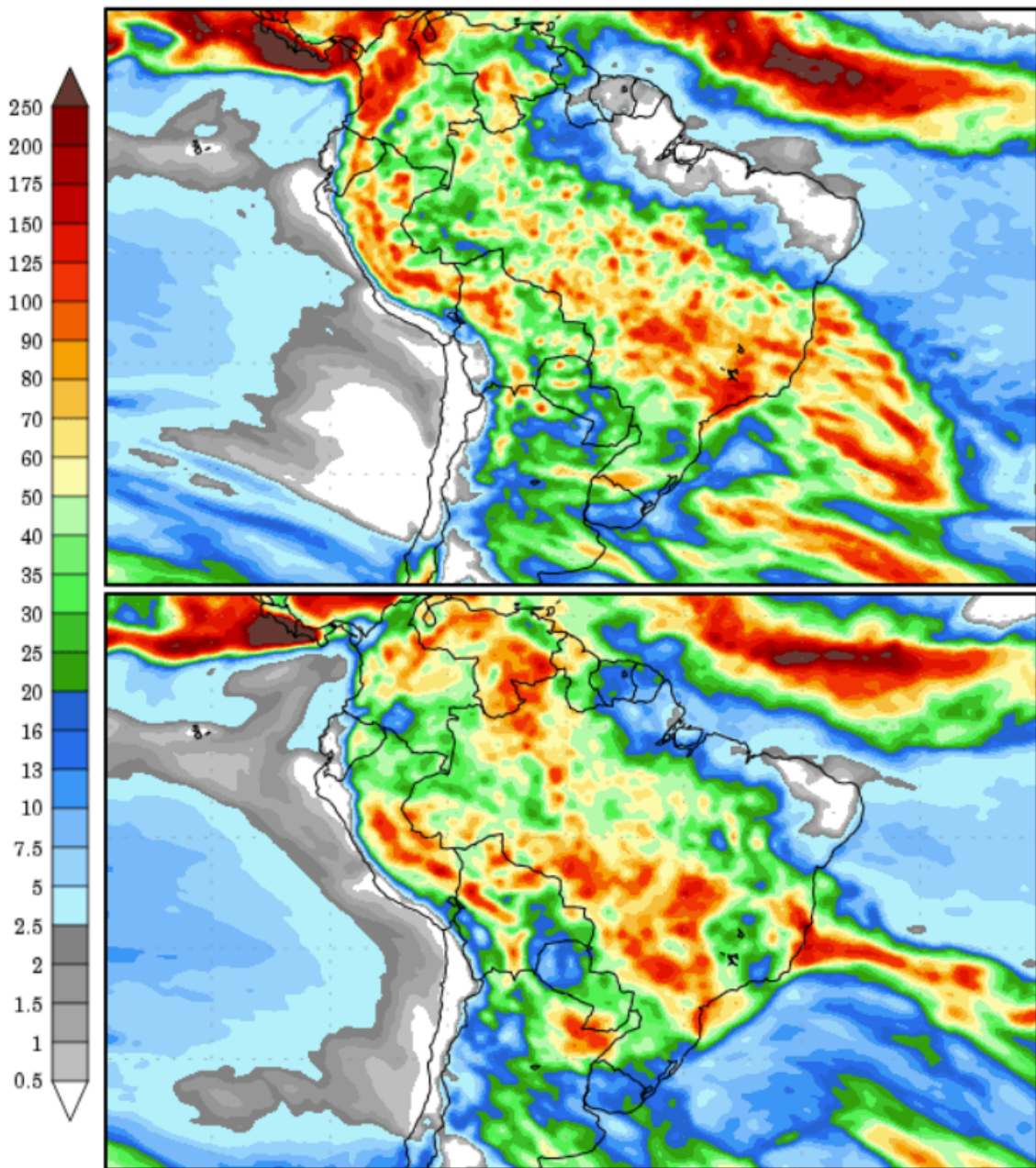
Figura 1. Precipitação acumulada prevista entre os dias 04 a 12 de novembro (imagem superior) e 12 a 20 de novembro de 2024 (imagem inferior). Fonte: COLA (Center for Ocean-Land-Atmosphere-Studies).
