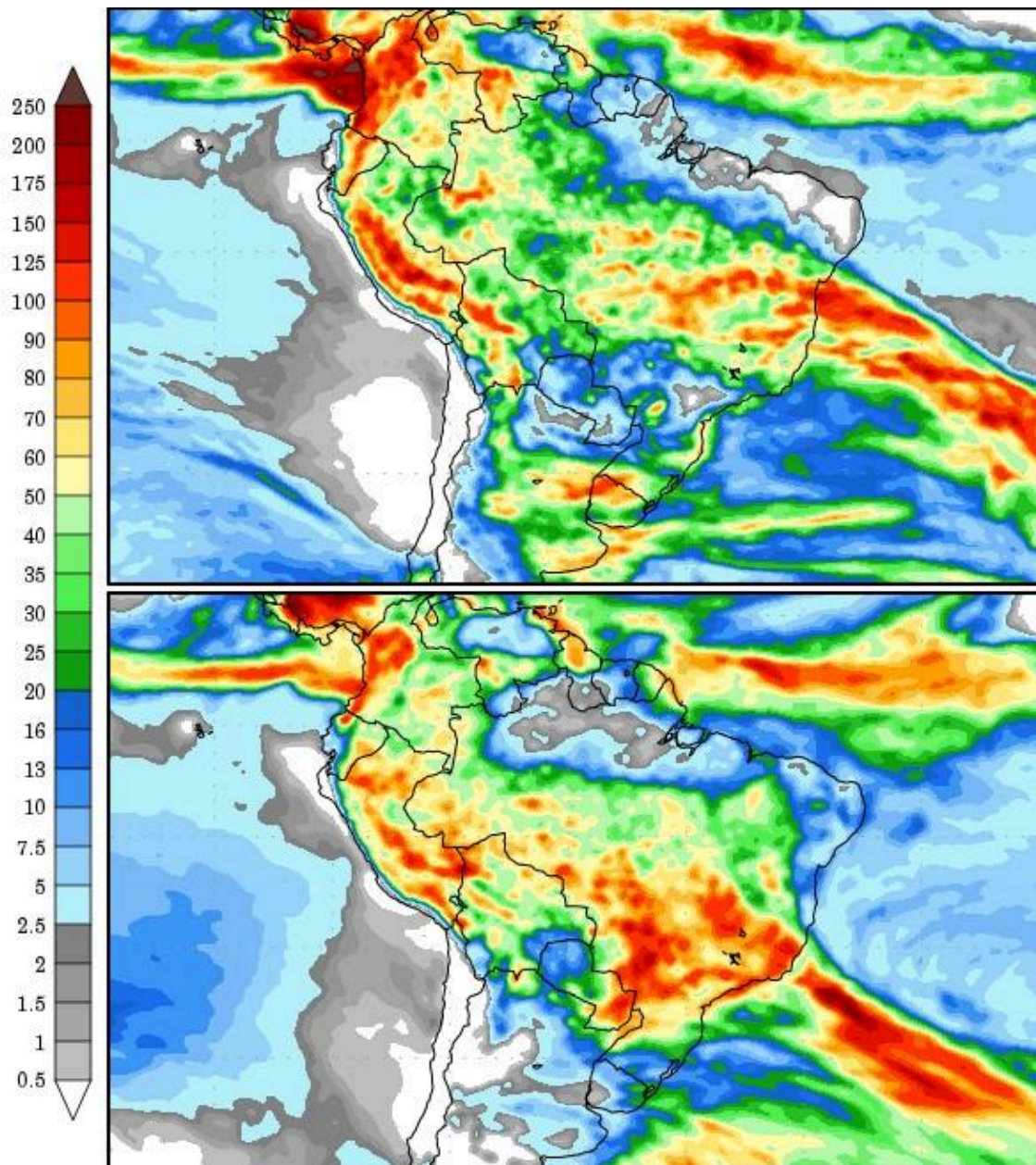
Figura 1. Precipitação acumulada prevista entre os dias 21 a 29 de novembro (imagem superior) e 29 de novembro a 07 de dezembro de 2024 (imagem inferior). Fonte: COLA (Center for Ocean-Land-Atmosphere-Studies).
