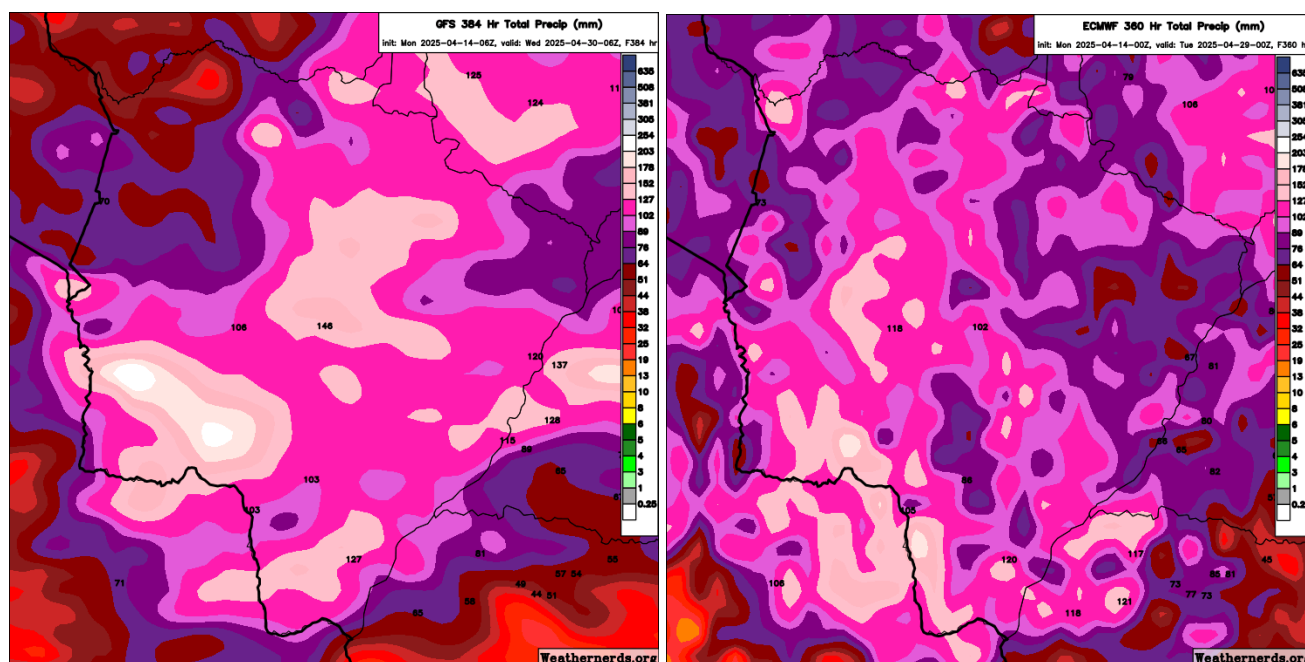
Figura 1. Precipitação acumulada prevista do modelo (a) GFS e (b) ECMWF para o período entre os dias 14 a 30 de abril de 2025. Fonte: Weathernerds.
