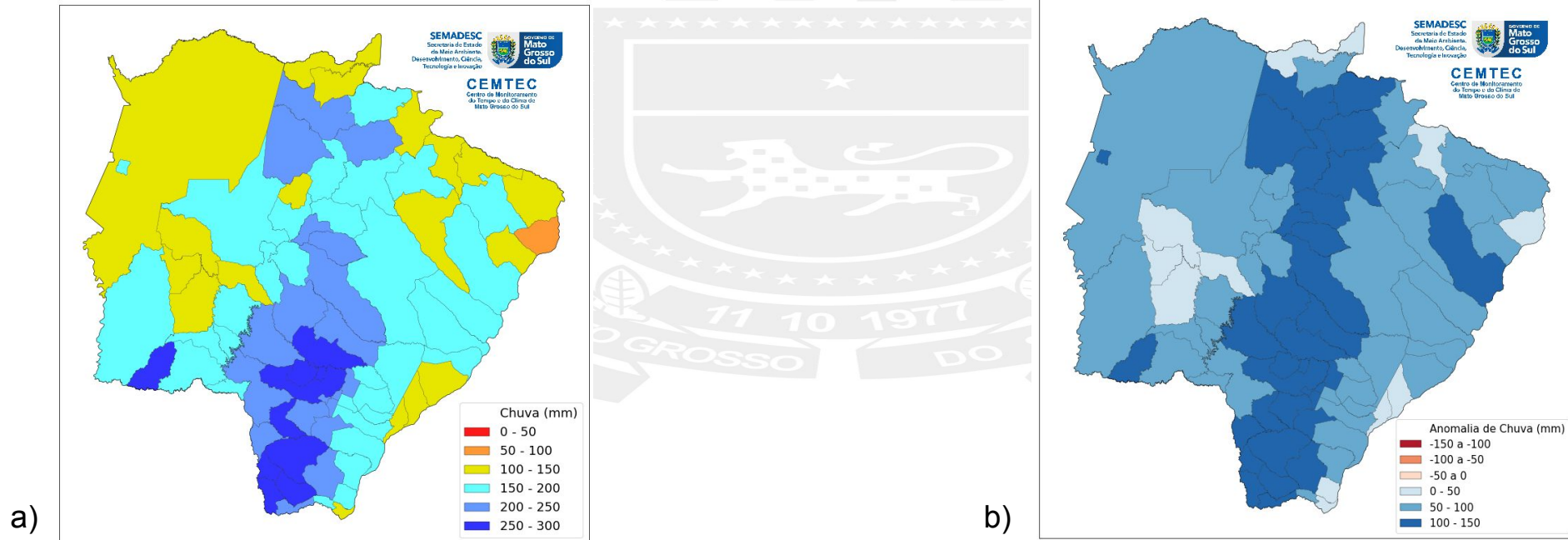
Figura 1. Precipitação acumulada (mm) (a) e Anomalia da Chuva (mm) (b) durante o mês de Abril de 2025. Fonte dos dados: MERGE/INPE. Processamento de dados: CEMTEC/SEMADESC.
