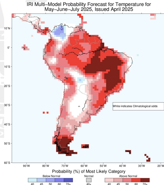
Figura 4. Média Histórica (a) e (b) Previsão probabilística em tercís da temperatura do ar para o trimestre de Maio-Junho-Julho (MJJ) de 2025. Fonte: INMET e IRI.
