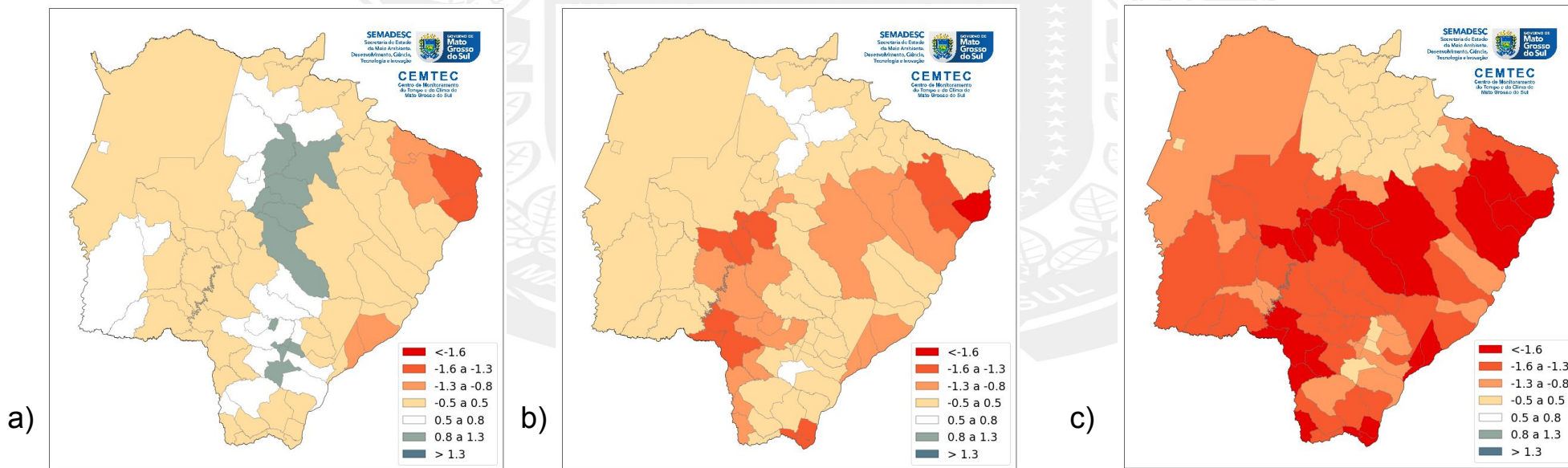
Figura 2. Índice Padronizado de Precipitação (SPI) na escala de (a) 3, (b) 6 e (c) 12 meses para o mês de abril de 2025. Fonte dos dados: MERGE/CPTEC/INPE. Processamento de dados:CEMTEC/SEMADESC.
