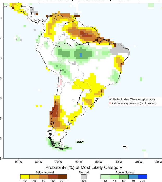
Figura 3. Média Histórica (a) e (b) Previsão probabilística em tercís da precipitação para o trimestre de Maio-Junho-Julho de 2025. Fonte: INMET e IRI.
