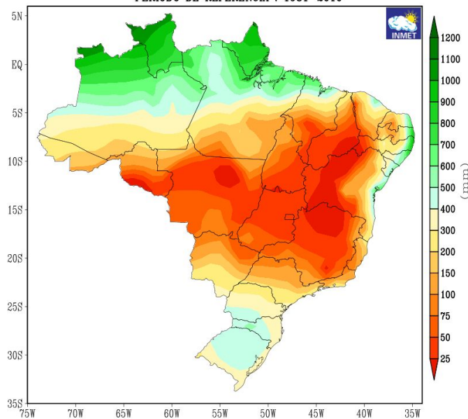
Figura 3. Média Histórica (a) e (b) Previsão probabilística em tercís da precipitação para o trimestre de Maio-Junho-Julho de 2025. Fonte: INMET e IRI.
