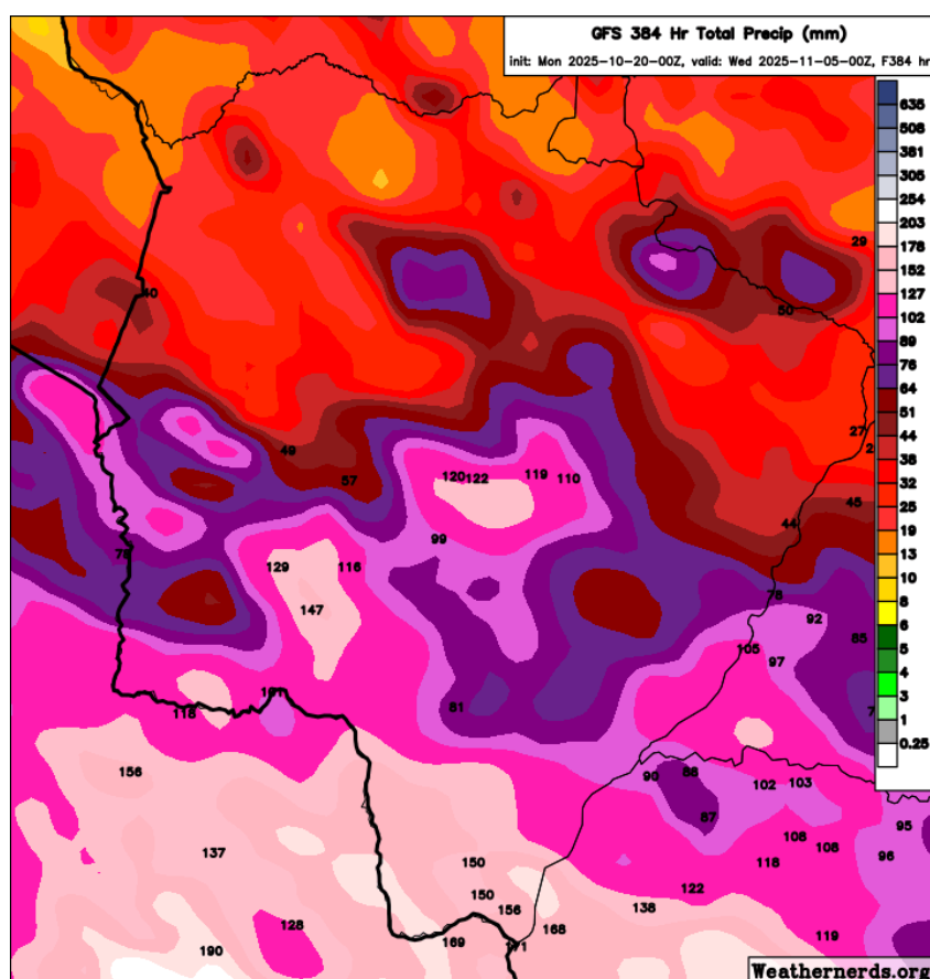
Figura 1. Precipitação acumulada prevista pelo modelo GFS para o período entre os dias 20 de outubro a 05 de novembro de 2025. Fonte: Weathernerds.
