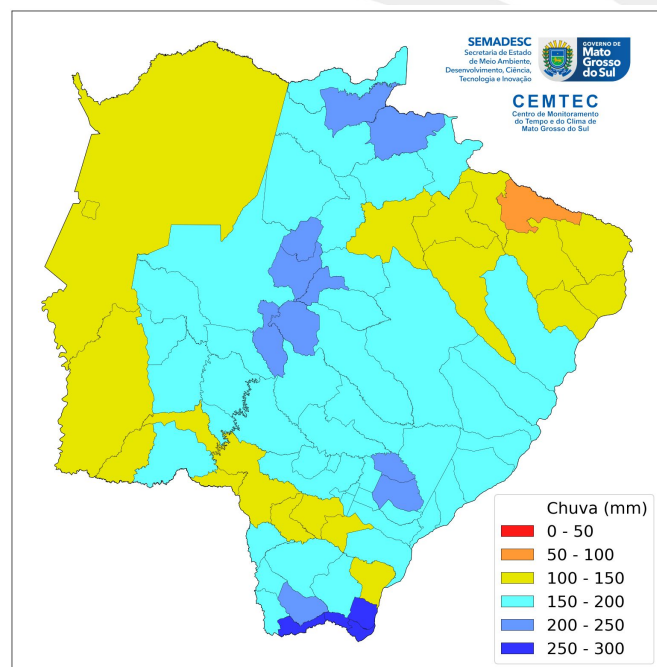
Figura 1. Precipitação acumulada (mm) (a) e Anomalia de Chuva (b) durante o mês de Dezembro de 2025. Fonte dos dados: MERGE/INPE. Processamento de dados: CEMTEC/SEMADESC.
