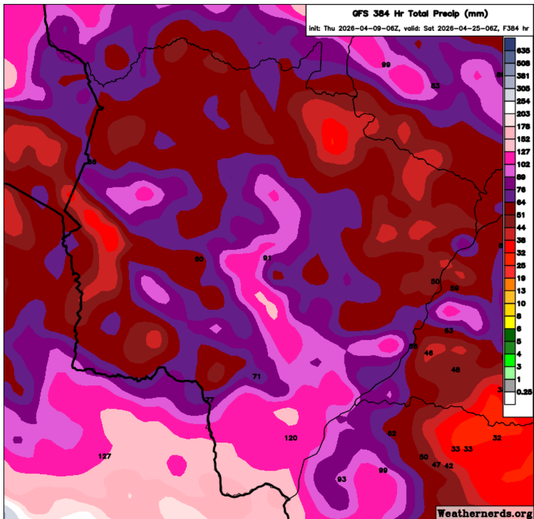
Figura 1. Precipitação acumulada prevista pelo modelo GFS para o período entre os dias 09 a 25 de abril de 2026. Fonte: Weathernerds.
