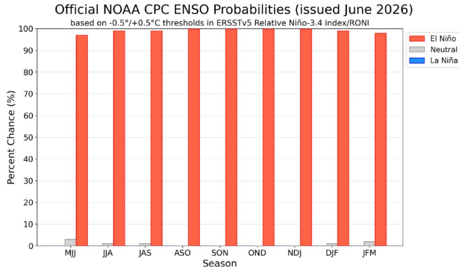
Figura 6. Previsão probabilística do El Niño Oscilação Sul (ENOS) trimestral. Fonte: CPC/IRI.
