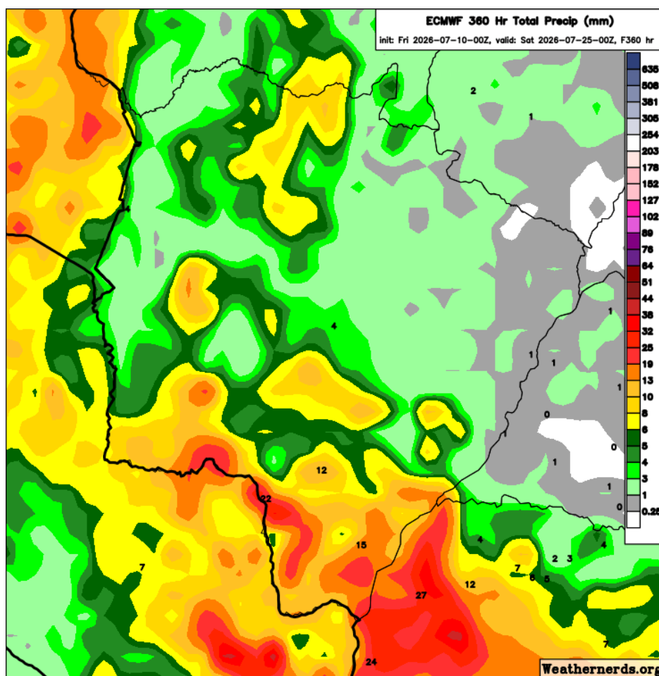
Figura 1. Precipitação acumulada prevista pelo modelo ECMWF para o período entre os dias 10 a 25 de julho de 2026. Fonte: Weathernerds.
