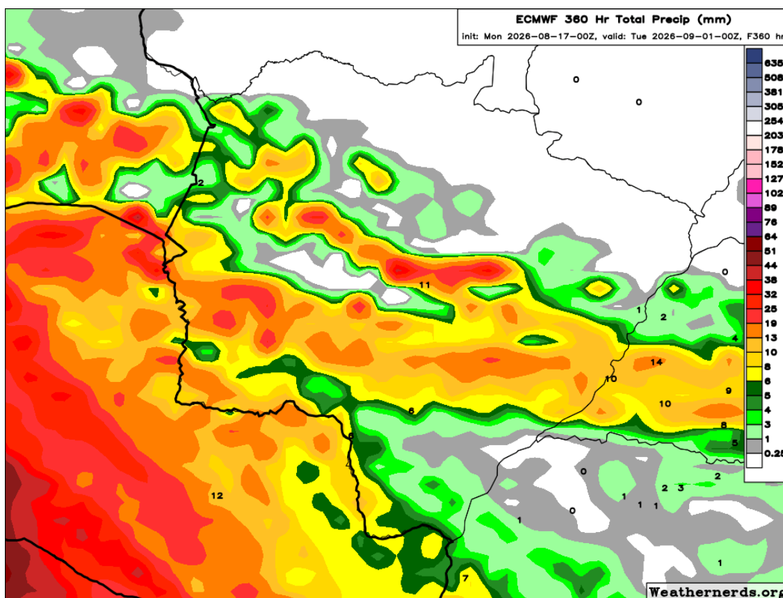
Figura 1. Precipitação acumulada prevista pelo modelo ECMWF para o período entre os dias 17 de agosto a 01 de setembro de 2026. Fonte: Weathernerds.
