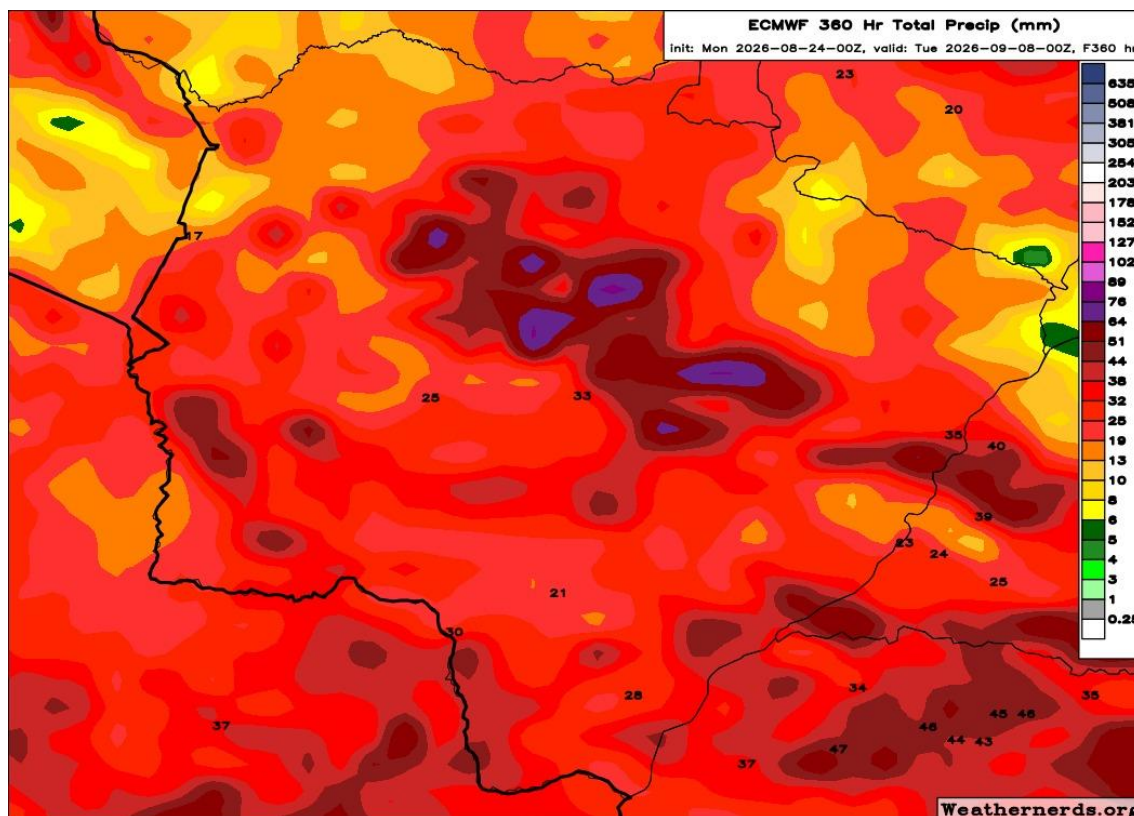
Figura 1. Precipitação acumulada prevista pelo modelo ECMWF para o período entre os dias 24 de agosto a 08 de setembro de 2026. Fonte: Weathernerds.
