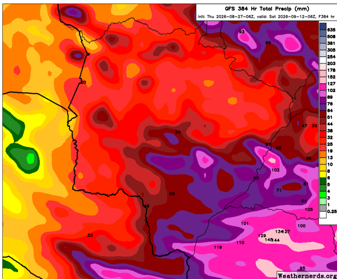
Figura 1. Precipitação acumulada prevista pelo modelo GFS para o período entre os dias 27 de agosto a 12 de setembro de 2026. Fonte: Weathernerds.
